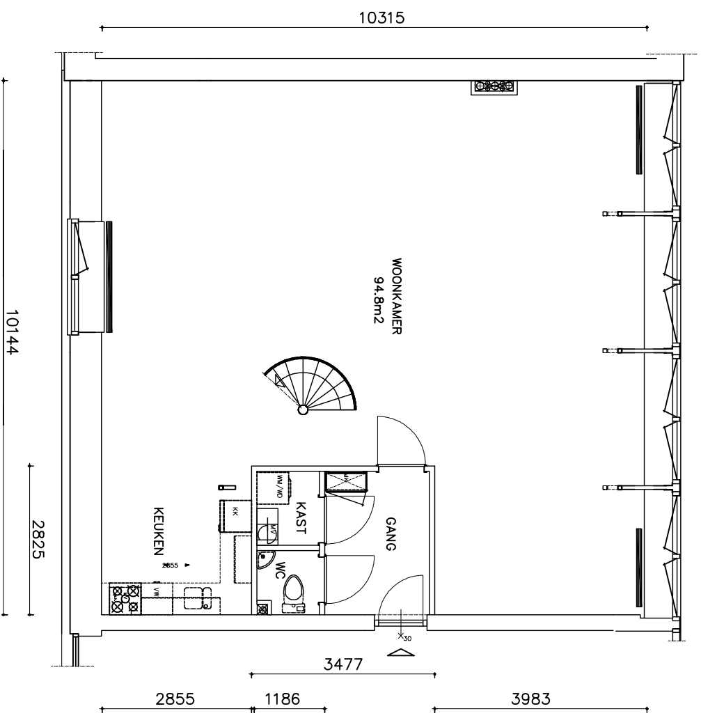
BOUWNUMMER-25 2e VERDIEPING
