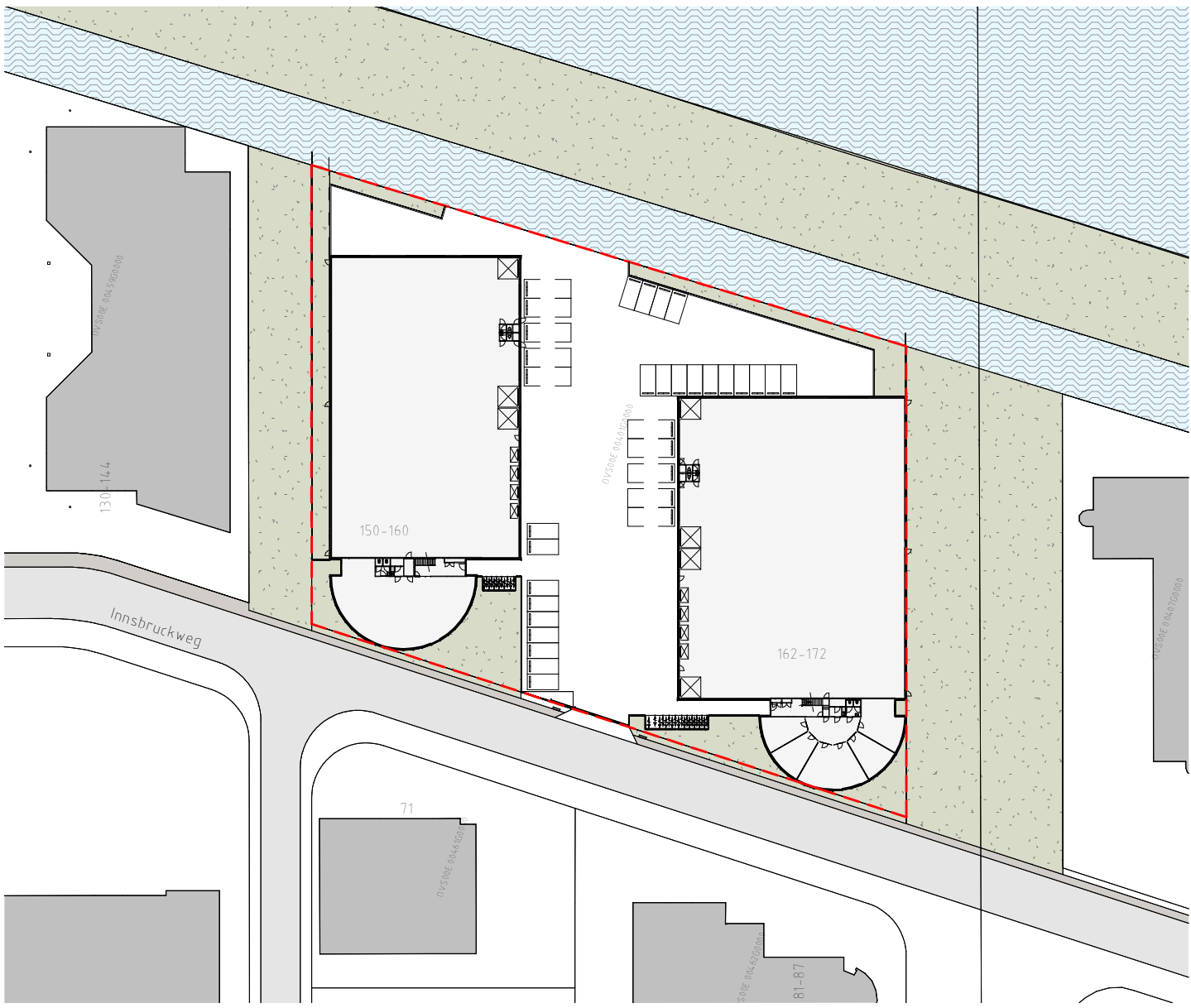
SITUATIE (1:1000)
