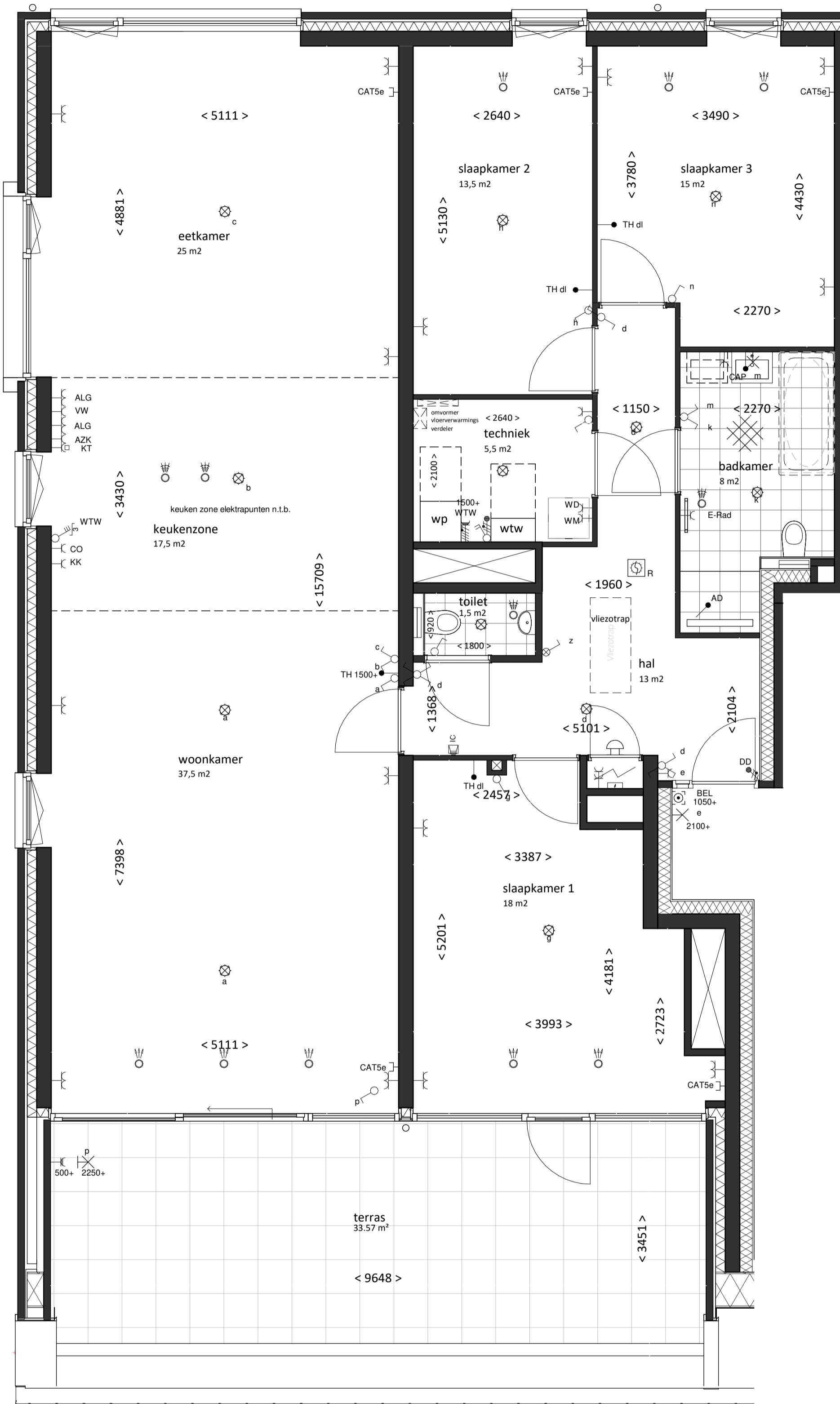
2e verdieping
